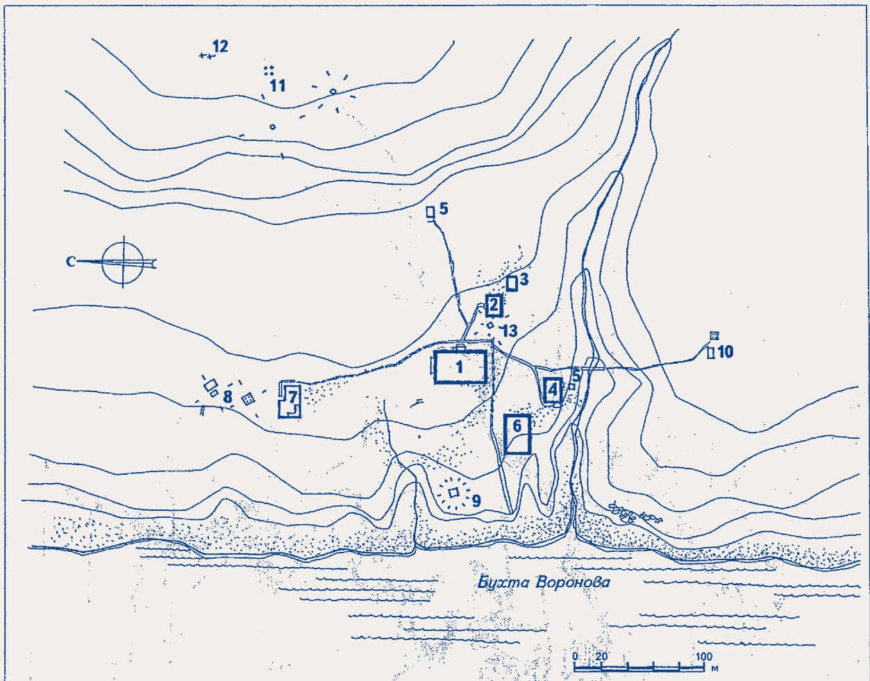
Полярная станция "Вайгач". Генплан.
